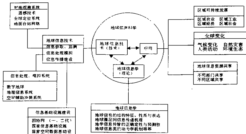
图 1 地球信息科学的科学体系
