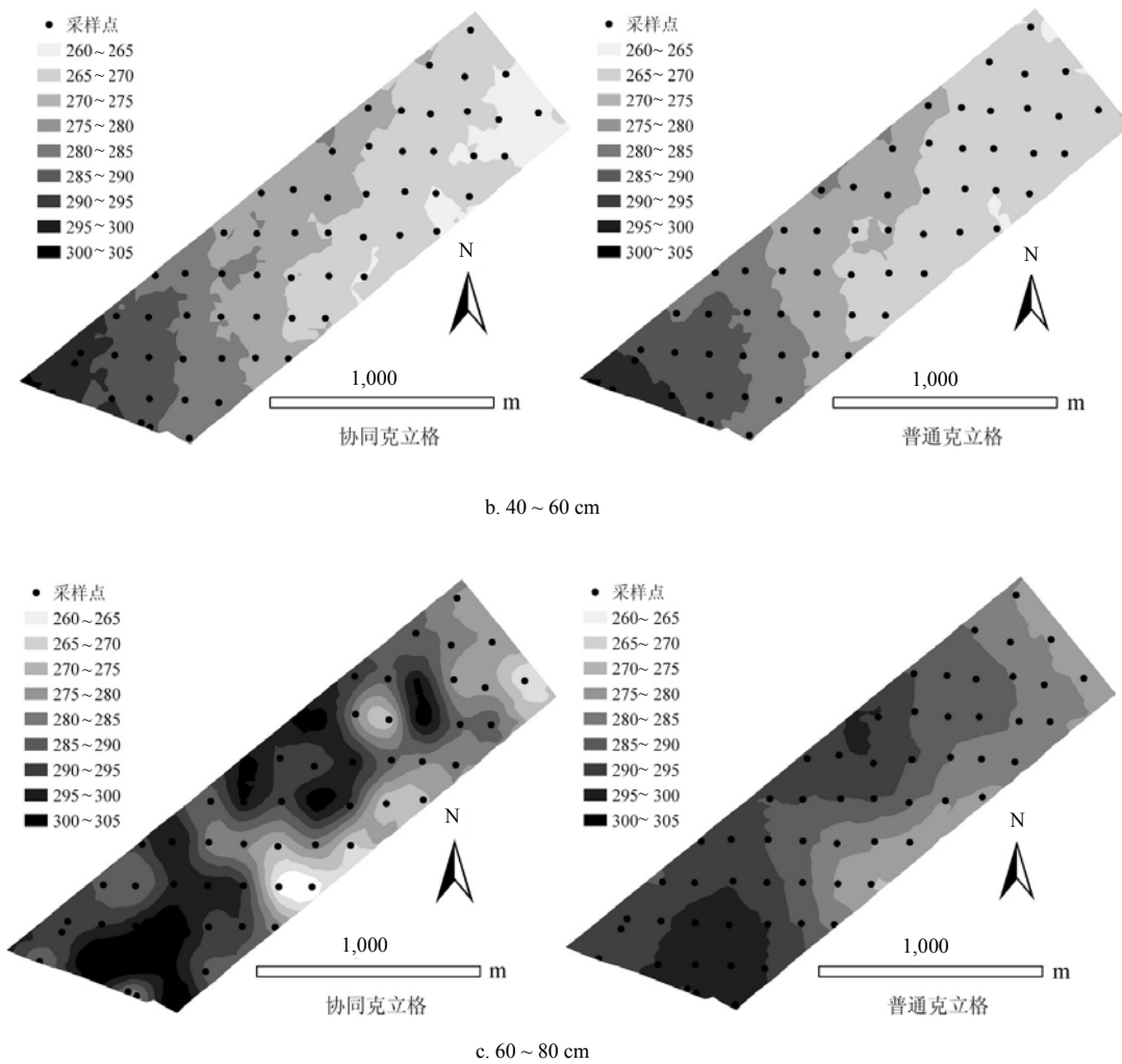
图 2 普通克立格和协同克立格对土壤含水量 (g/kg) 插值的空间分布图
