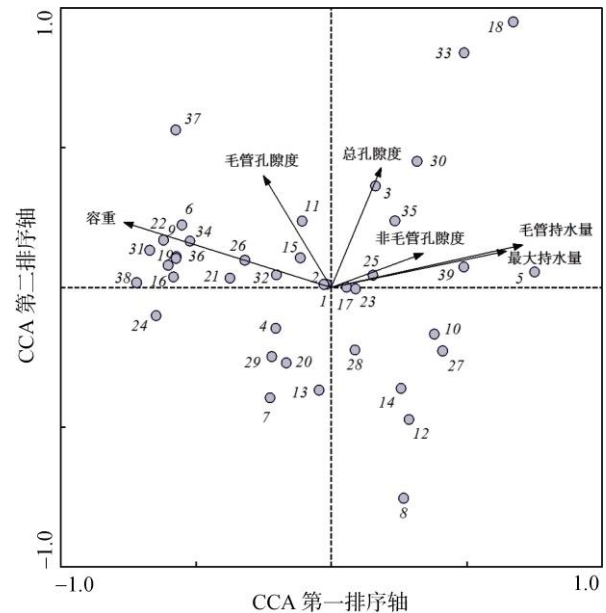
(图中圆圈代表各物种在环境梯度上的最优分布位置, 数字为物种代码(表 2 所示); 箭头方向代表某个环境因子与排序轴的正负相关性, 箭头连线长短代表环境因子与物种分布之间关系的强弱(线越长则相关性越大), 箭头连线与排序轴夹角代表环境因子与排序轴相关性的大小(夹角越小则相关性越大); 下同)
